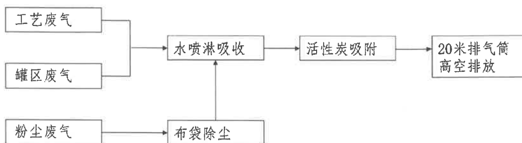
图 4.2-1 厂区废气处理流程图
