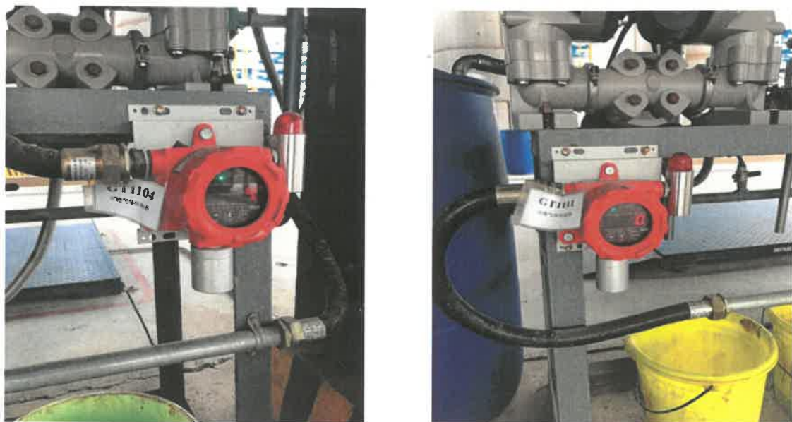
图 4.1-2 可燃及有毒气体监控装置图
